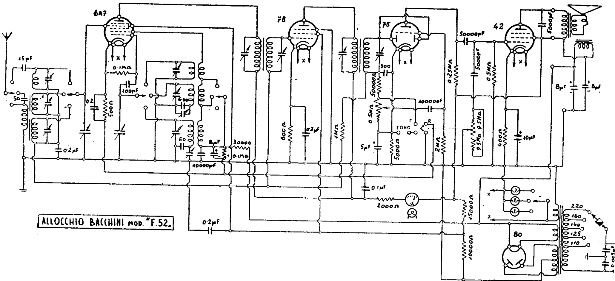
ALLOCCIO, BACCHINI e Co — Mod. F 52 M, Mod F 52 R e Mod F 52 G - Produzione 1937 Media frequenza 425 kHz.
